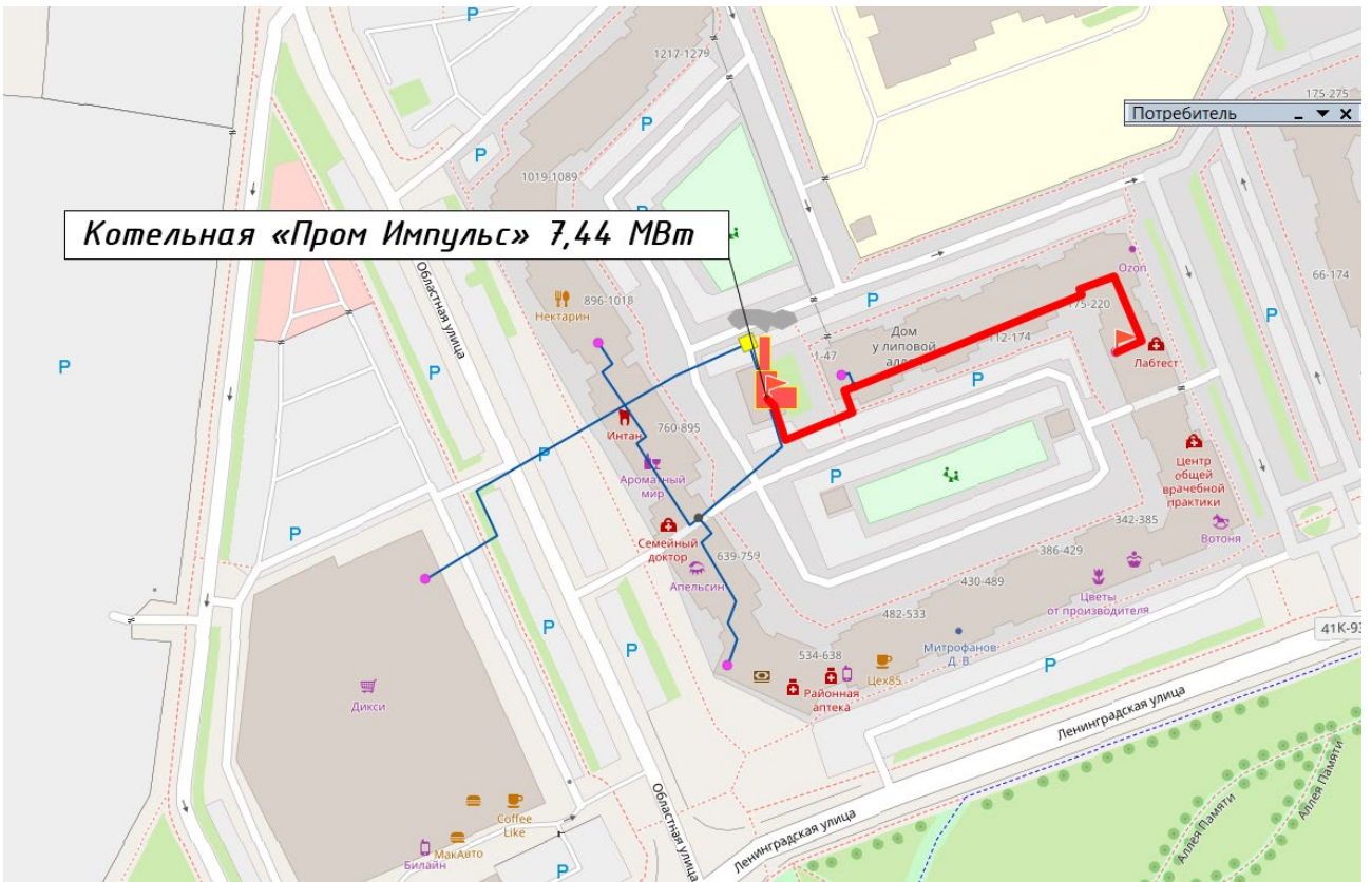
Рисунок 45. Путь построения пьезометрического графика от котельной 7,44 МВт
