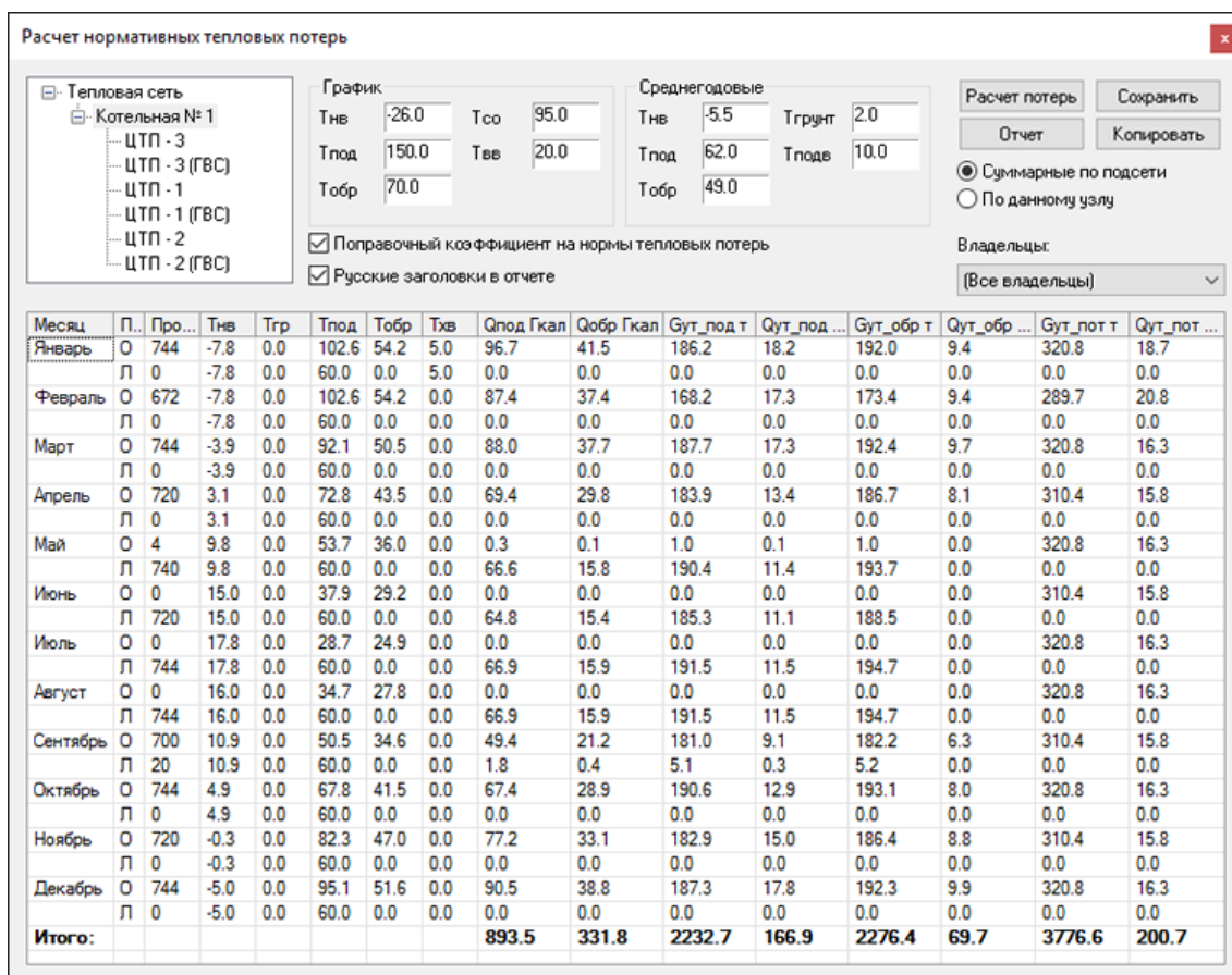
Рисунок 24. Результаты расчета потерь тепловой энергии через изоляцию и с утечками теплоносителя
