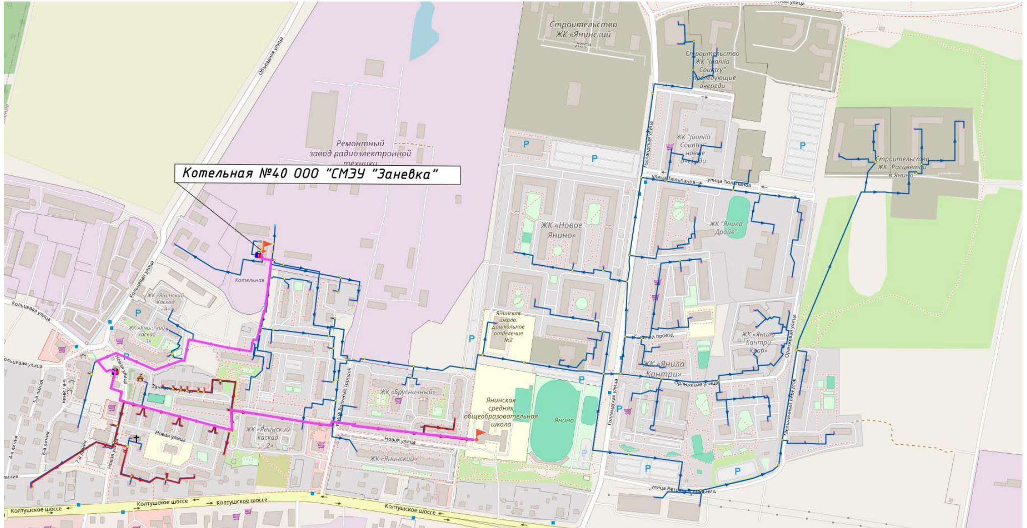
Рисунок 30. Путь построения пьезометрического графика от ЦТП система -95/70С
