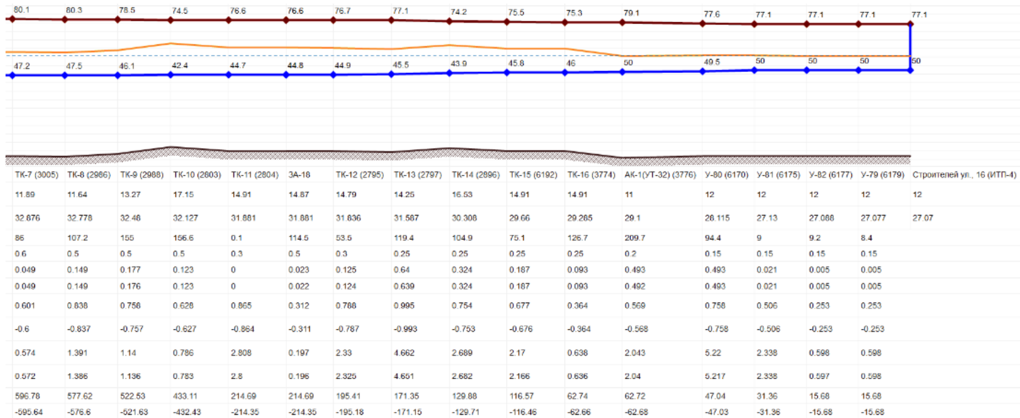
Рисунок 34. Пьезометрический график от Правобережной ТЭЦ-5(часть 2)
