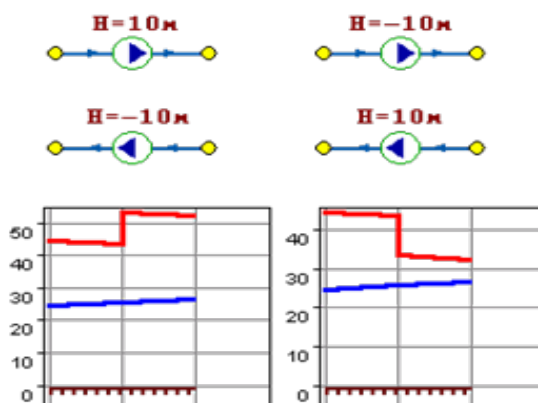
Рисунок 16. Пьезометрические графики
