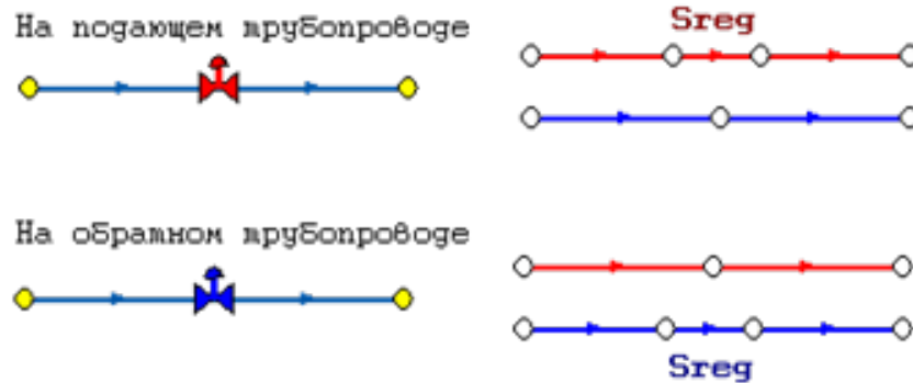
Рисунок 18. Дросселирующие устройства
