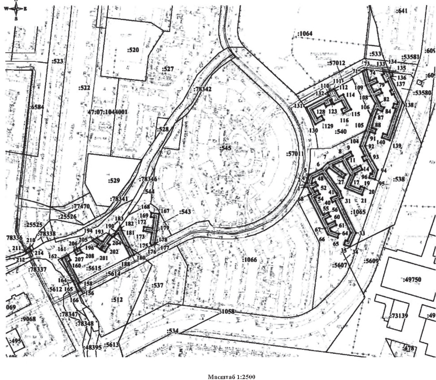
Система координат МСК 47 зона 2 Общая площадь публичного сервитута: 6795 кв.м
