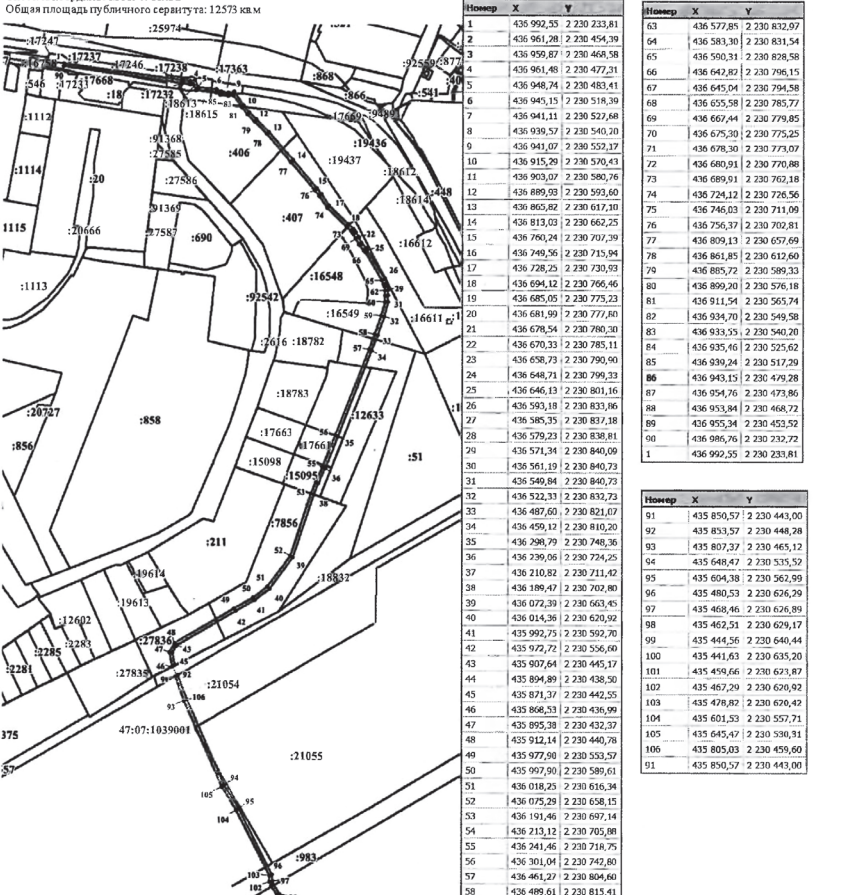
Система координат МСК 47 зона 2 Общая площадь публичного сервитута: 12573 кв.м
